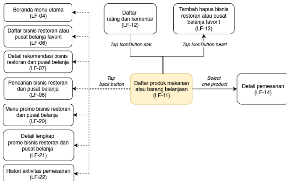
Gambar C.10. Diagram navigasi layar untuk halaman daftar produk makanan atau barang belanjaan
