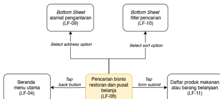
Gambar C.8. Diagram navigasi layar untuk halaman pencarian bisnis restoran dan pusat belanja
