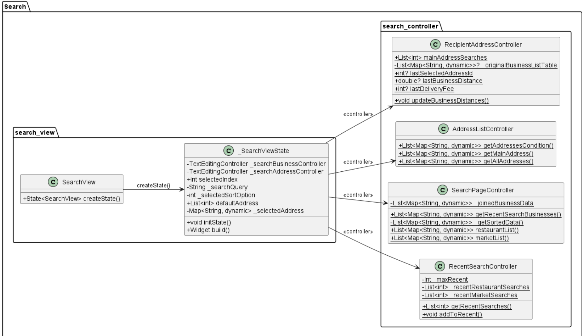
Gambar M.8. Class diagram untuk halaman pencarian bisnis restoran dan pusat belanja
