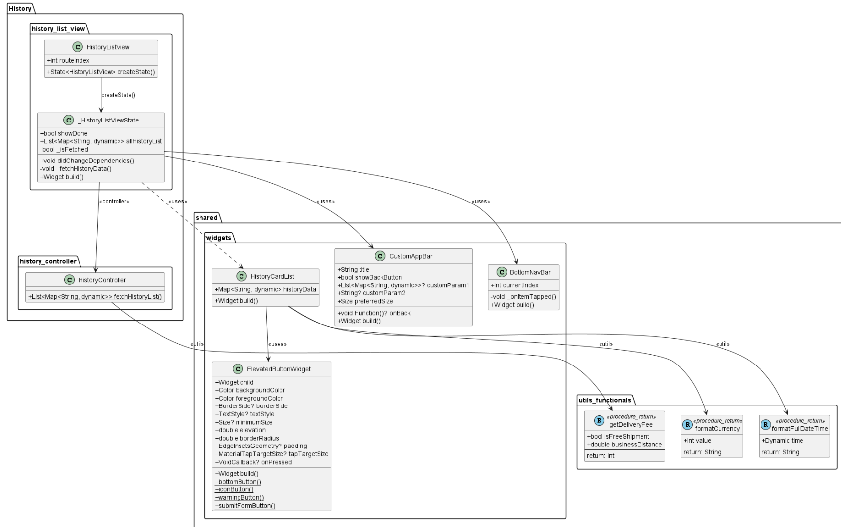
Gambar M.21. Class diagram untuk halaman histori aktivitas pemesanan
