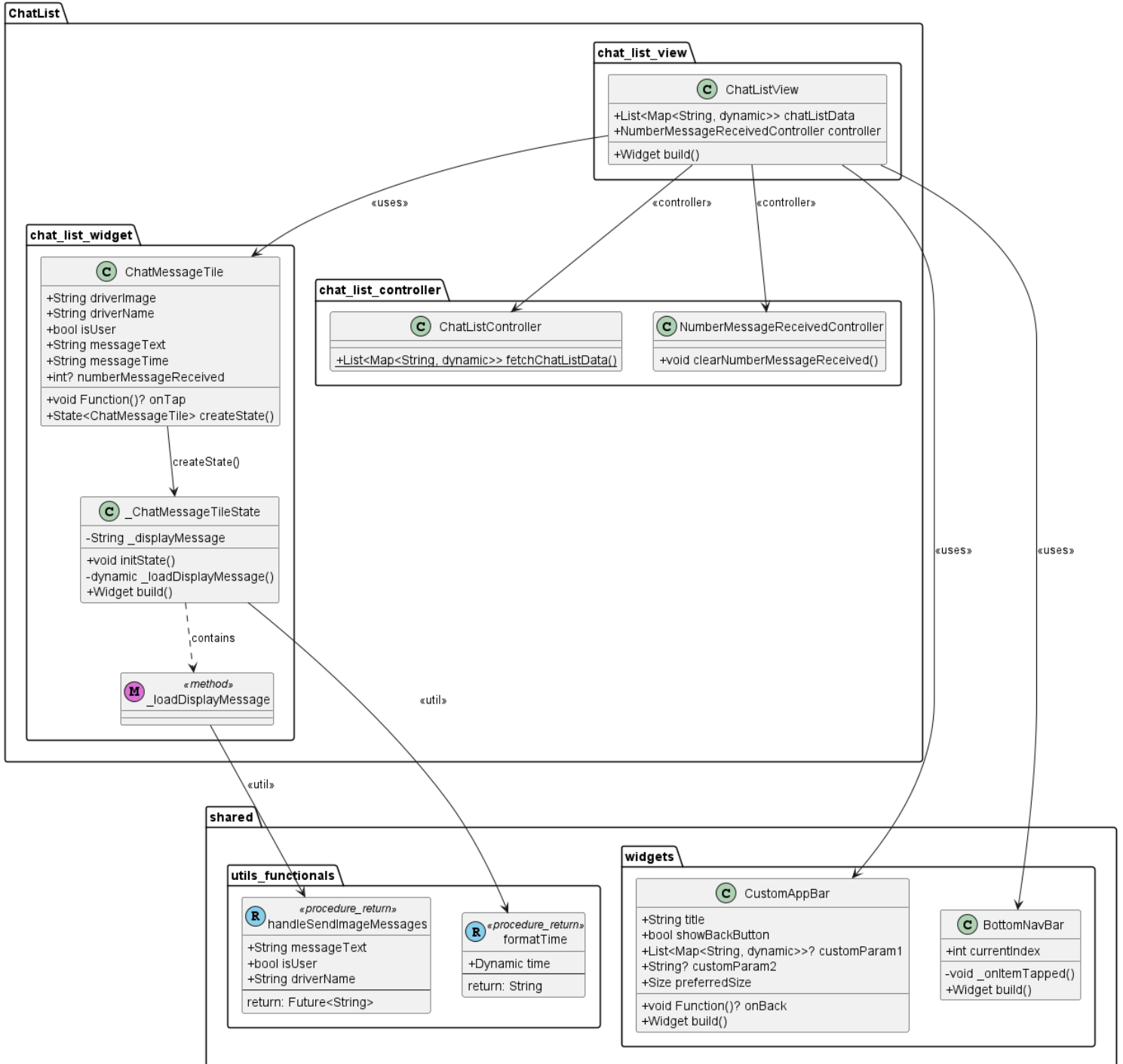
Gambar M.26. Class diagram untuk halaman daftar keseluruhan kontak
