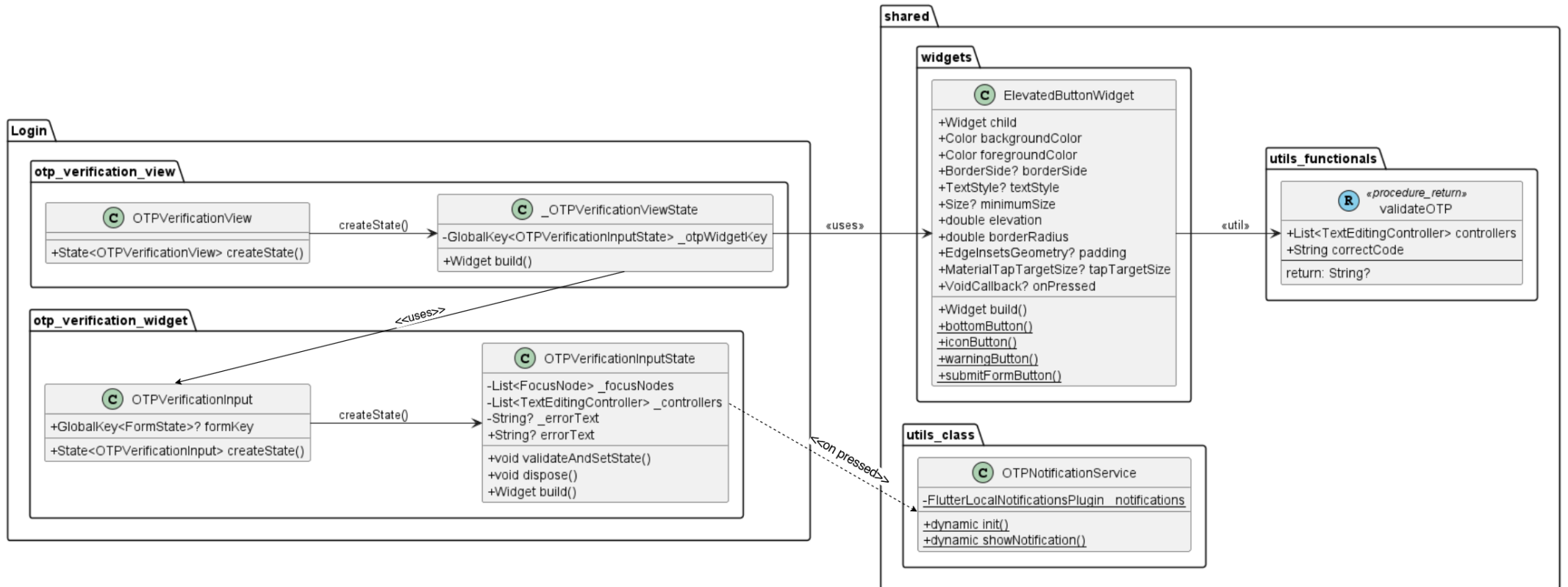
Gambar M.3. Class diagram untuk halaman verifikasi OTP dengan nomor telepon
