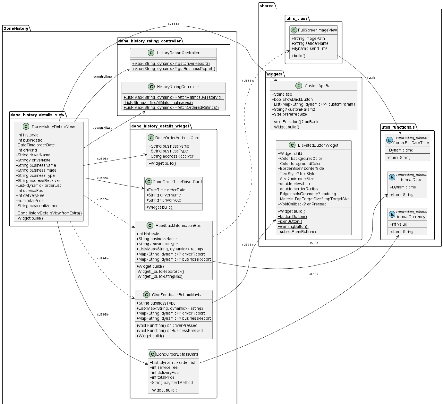
Gambar M.22. Class diagram untuk halaman detail aktivitas pemesanan sebelumnya
