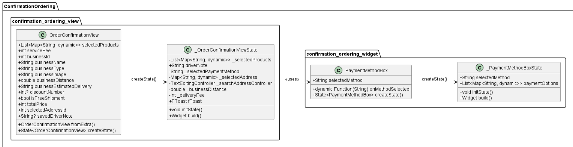
Gambar M.18. Class diagram untuk bottom sheet pemilihan metode pembayaran
