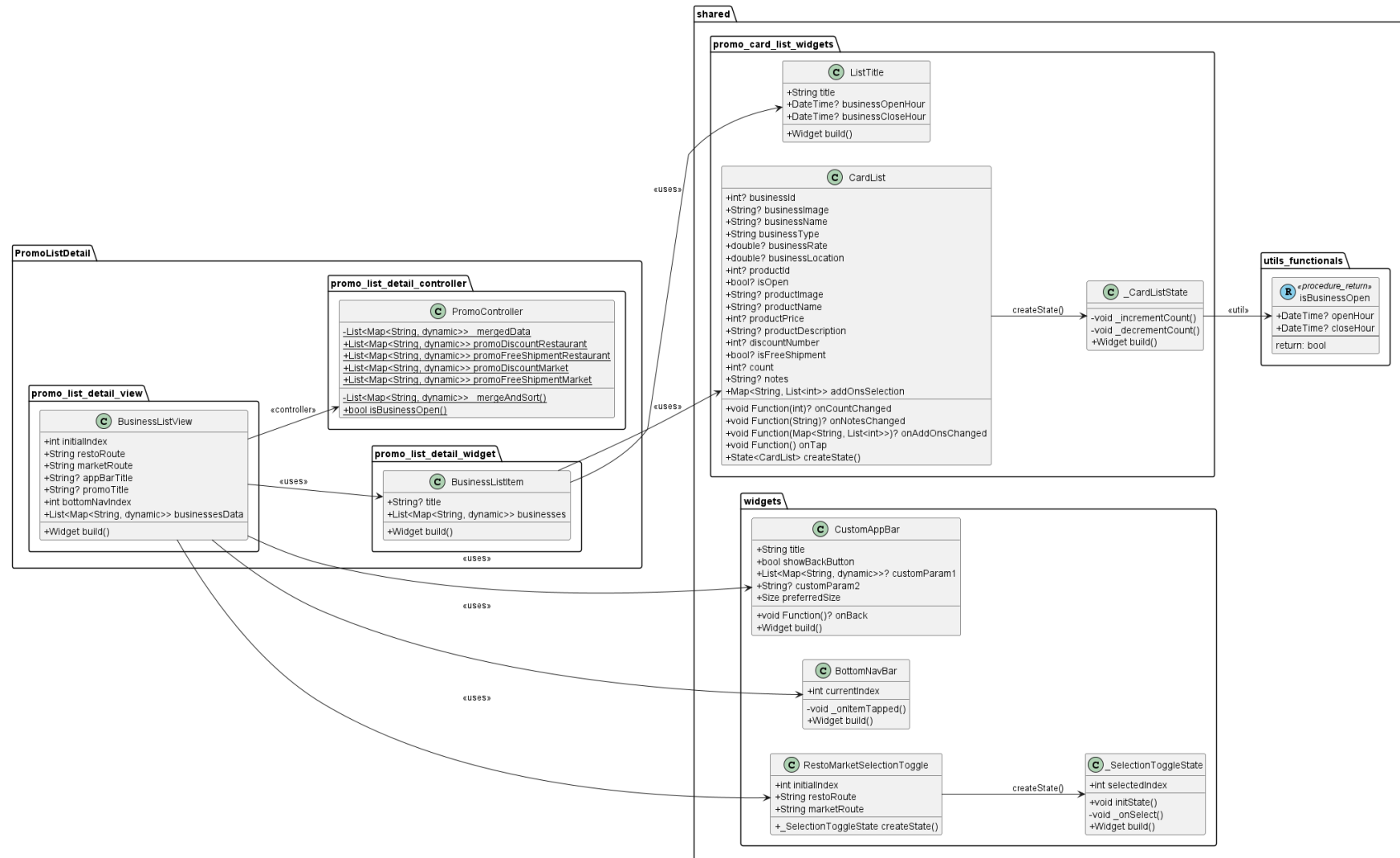
Gambar M.20. Class diagram untuk halaman detail lengkap promo bisnis restoran dan pusat belanja
