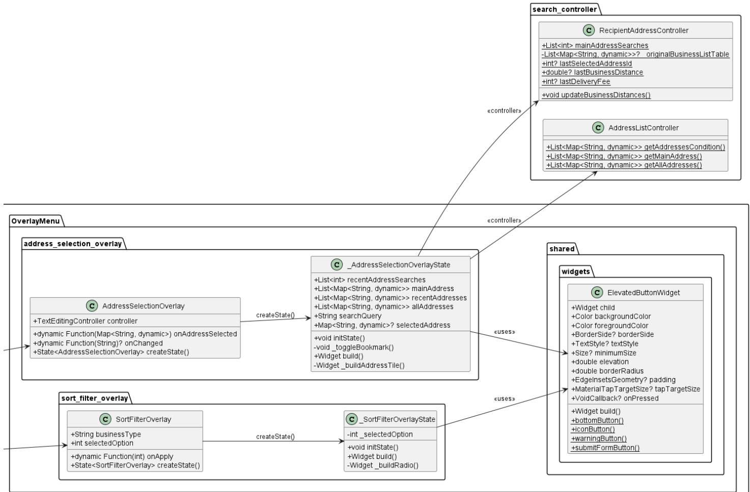
Gambar M.9. Class diagram untuk bottom sheet alamat pengantaran dan sort pencarian
