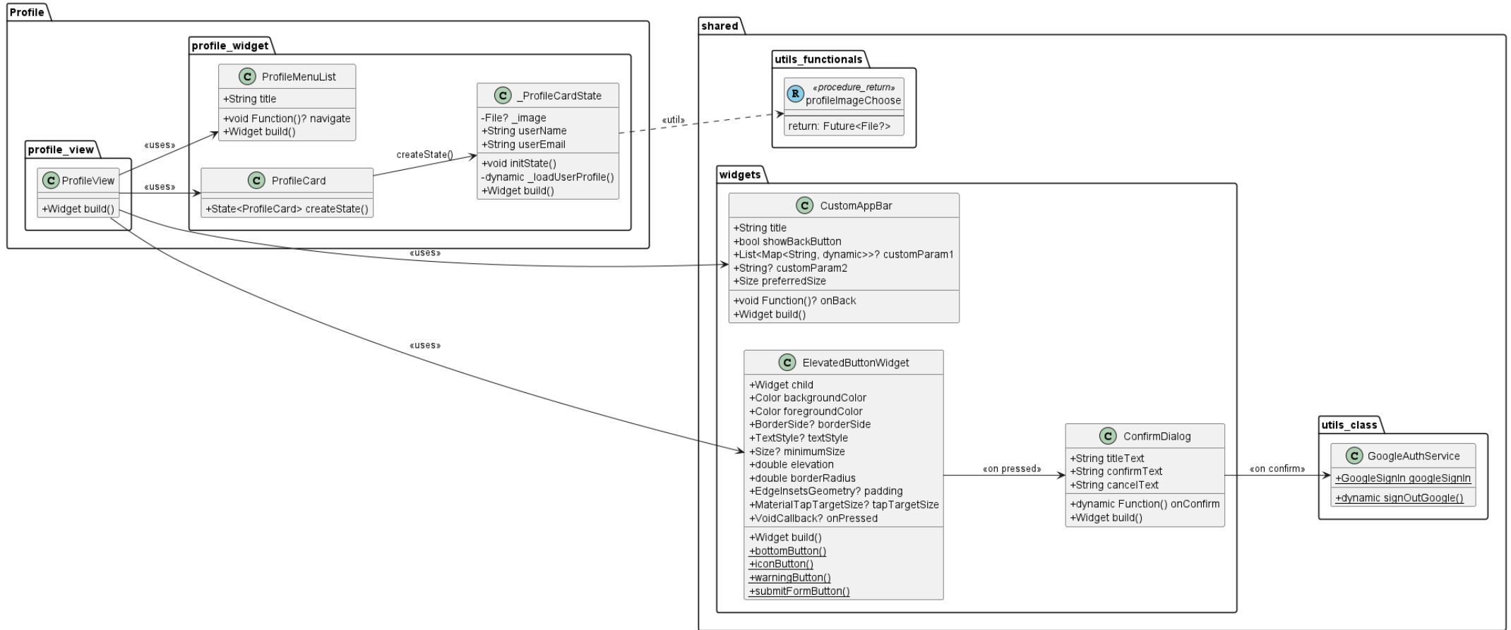
Gambar M.5. Class diagram untuk halaman profil pribadi
