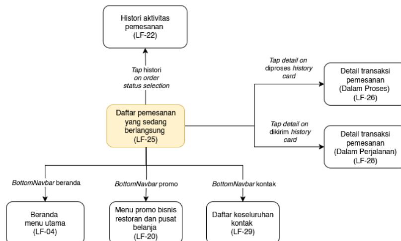
Gambar C.22. Diagram navigasi layar untuk halaman daftar pemesanan yang sedang berlangsung
