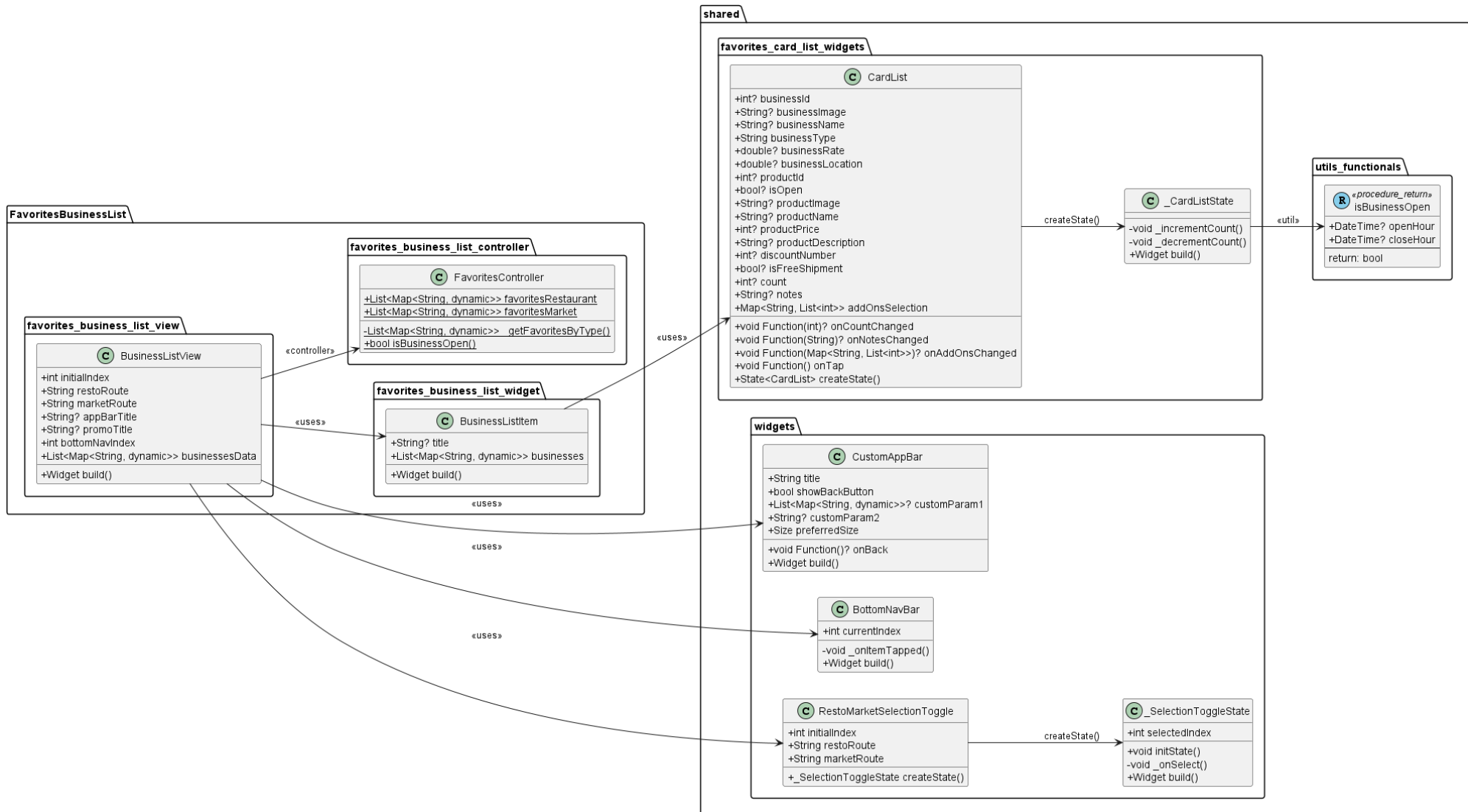
Gambar M.6. Class diagram untuk halaman daftar bisnis restoran dan pusat belanja favorit
