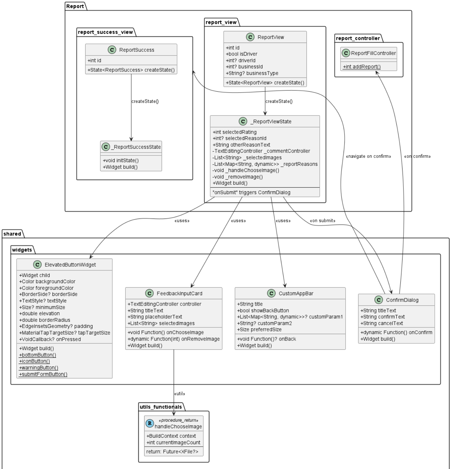
Gambar M.28. Class diagram untuk halaman pelaporan
