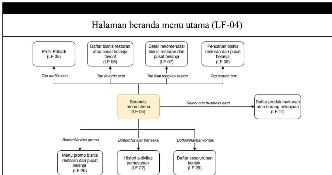
Gambar C.4. Diagram navigasi layar untuk halaman beranda menu utama
