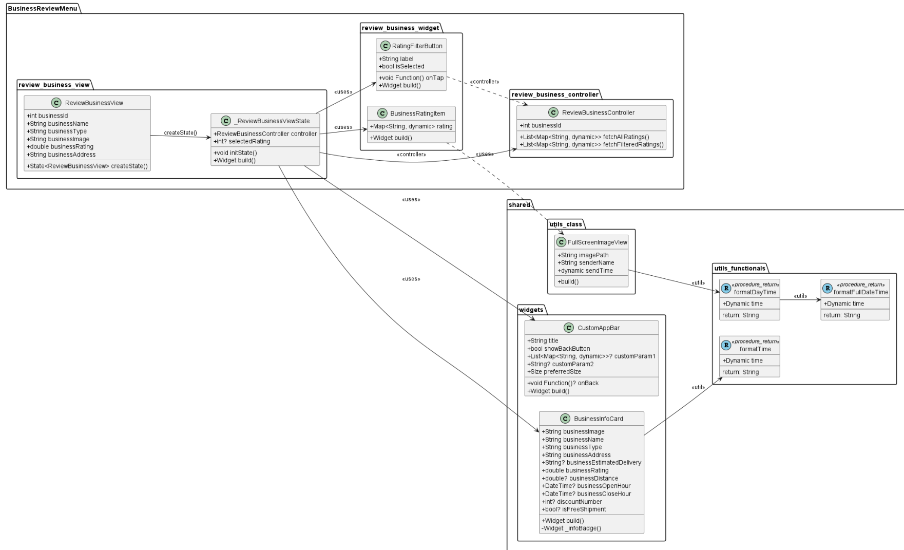
Gambar M.11. Class diagram untuk halaman daftar rating dan komentar
