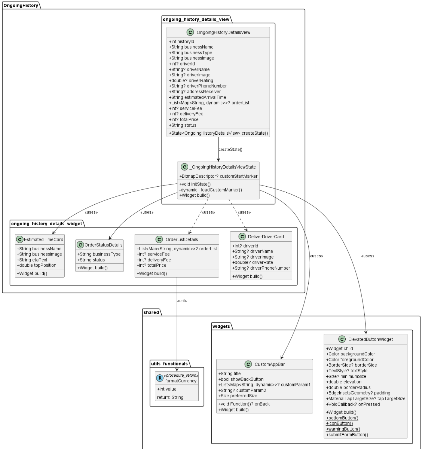
Gambar M.24. Class diagram untuk halaman keseluruhan detail transaksi pemesanan
