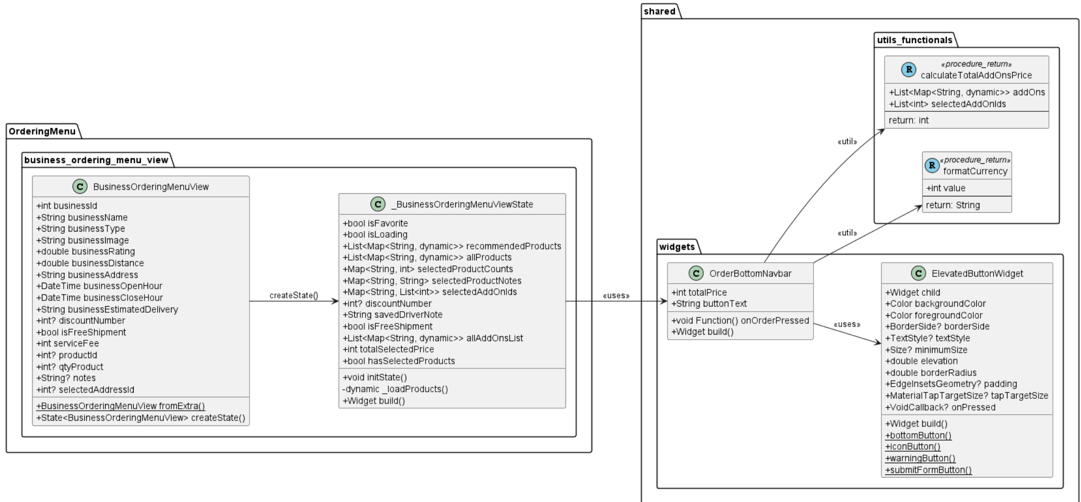
Gambar M.14. Class diagram untuk bottom bar konfirmasi pemesanan
