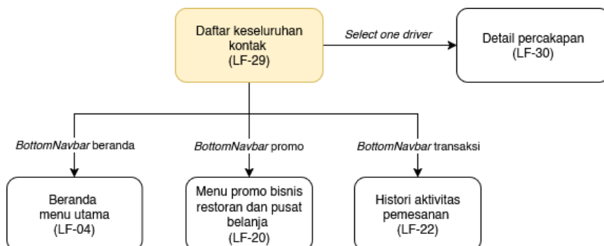
Gambar C.26. Diagram navigasi layar untuk halaman daftar keseluruhan kontak
