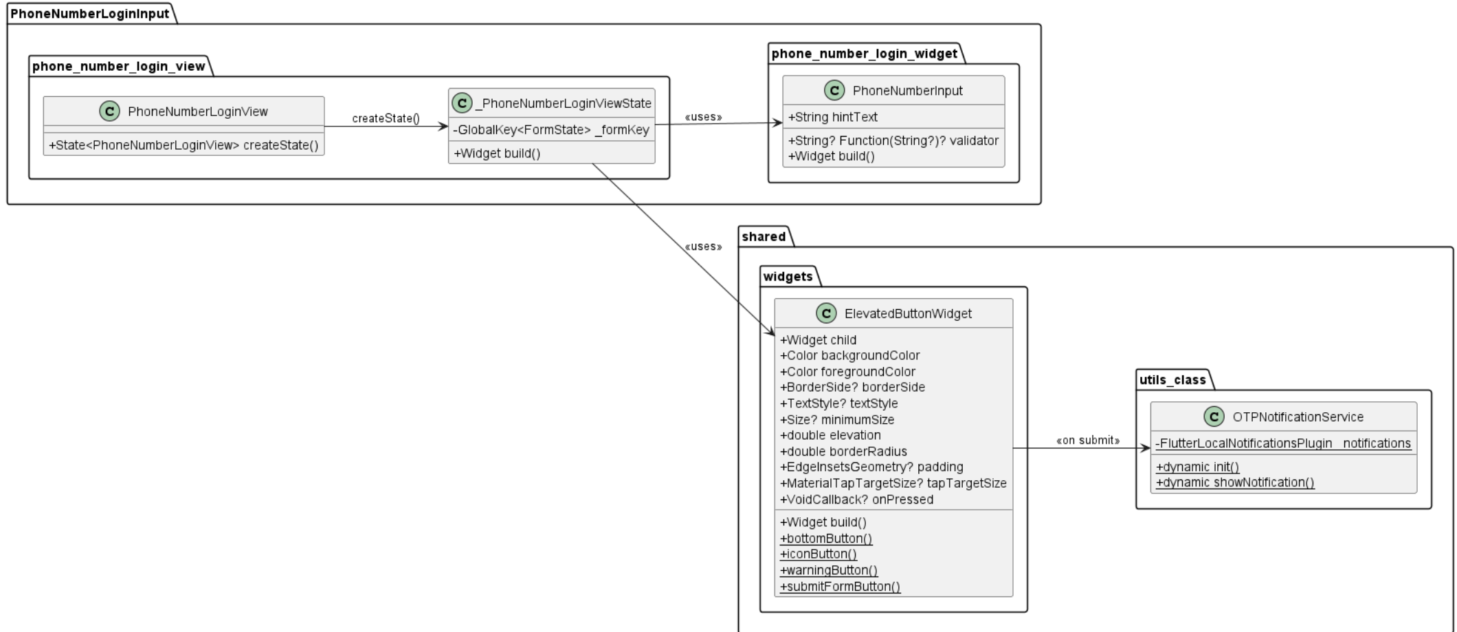
Gambar M.2. Class diagram untuk halaman login dengan nomor telepon
