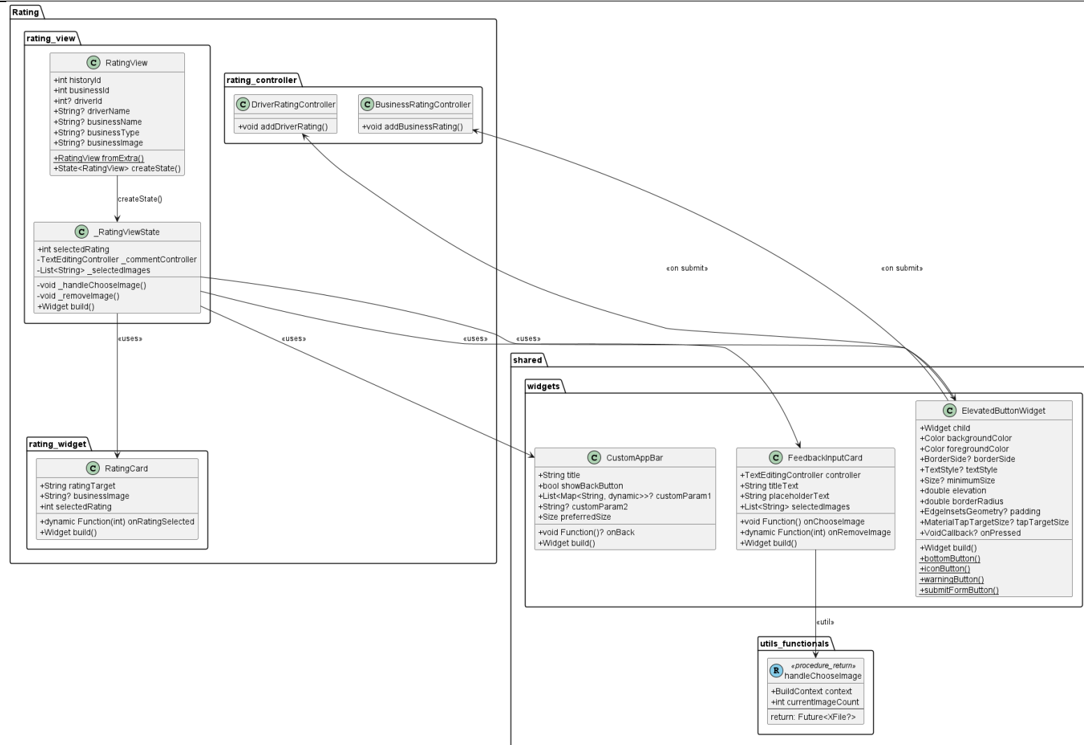
Gambar M.23. Class diagram untuk halaman pemberian rating dan komentar
