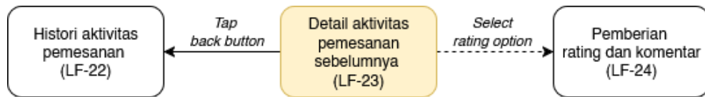
Gambar C.20. Diagram navigasi layar dari halaman detail aktivitas pemesanan sebelumnya
