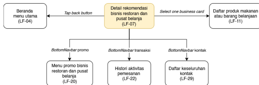
Gambar C.7. Diagram navigasi layar untuk halaman detail rekomendasi restoran dan pusat belanja
