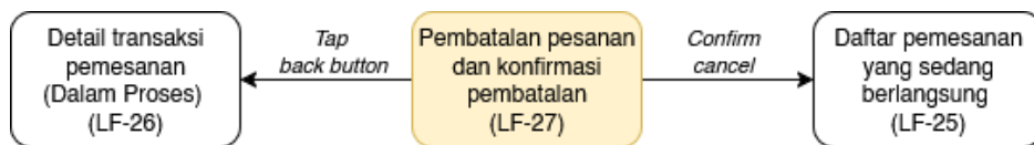
Gambar C.24. Diagram navigasi layar untuk halaman pembatalan pesanan dan dialog konfirmasi pembatalan
