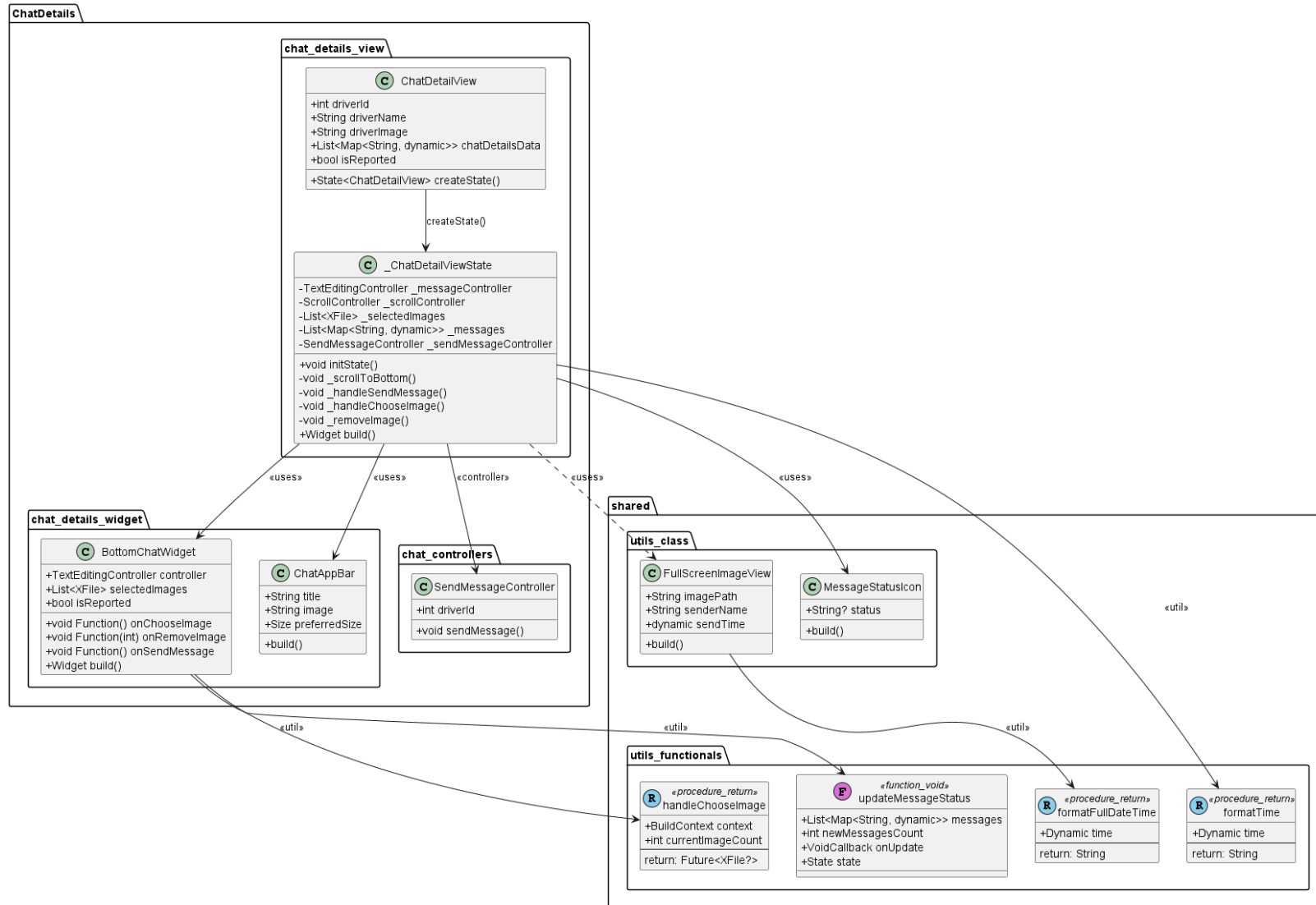
Gambar M.27. Class diagram untuk halaman detail percakapan
